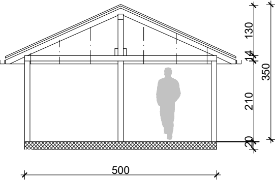
PRESJEK A
