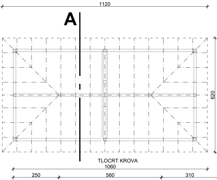
TLOCRT KROVIŠTA
