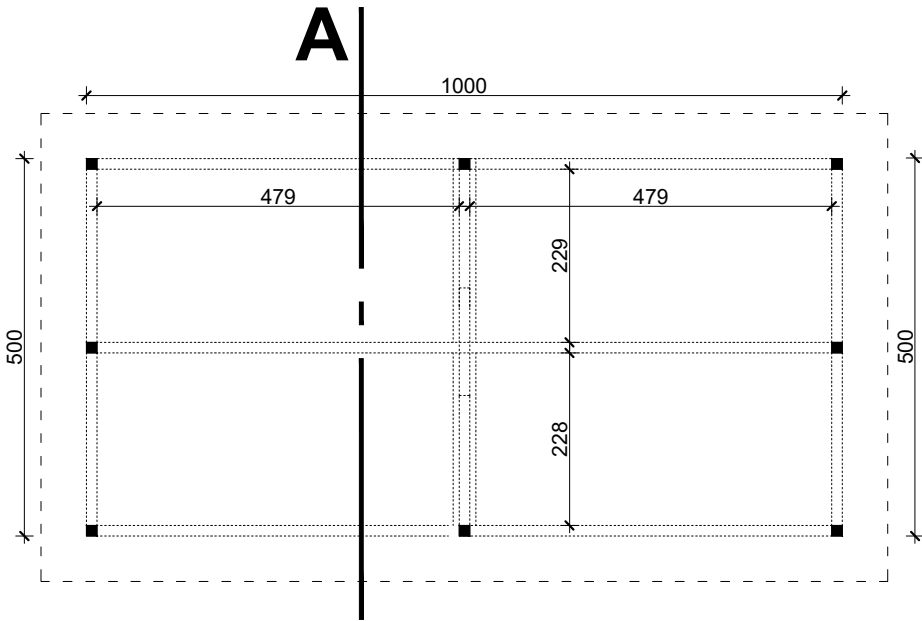
TLOCRT PRIZEMLJA
