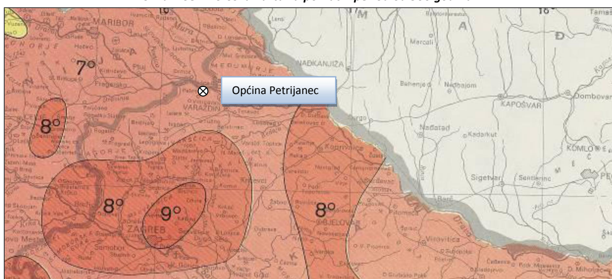
Slika 2. Seizmološka karta za povratni period od 500 godina
