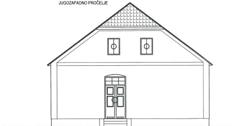
JUGOZAPADNO PROČELJE
