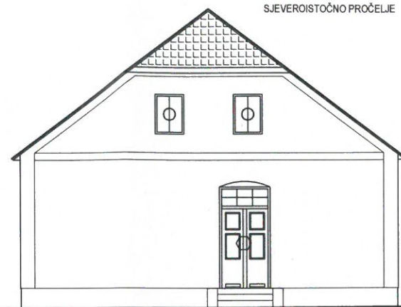
SJEVEROISTOČNO PROČELJE
